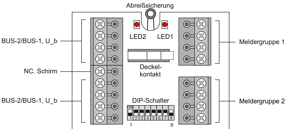
Die Anschlussklemmen sind steckbar
